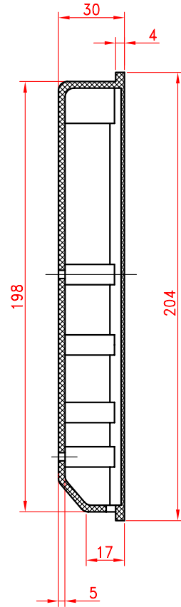
SECTION A-A
